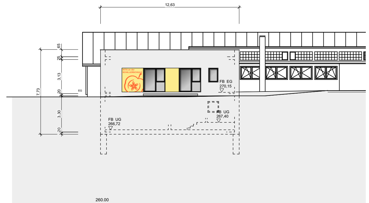
ANSICHT OST
