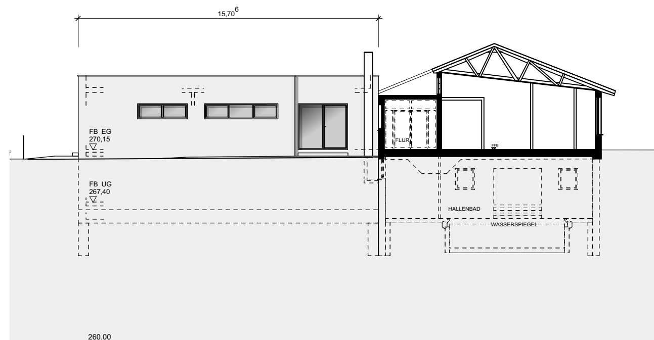
ANSICHT NORD
