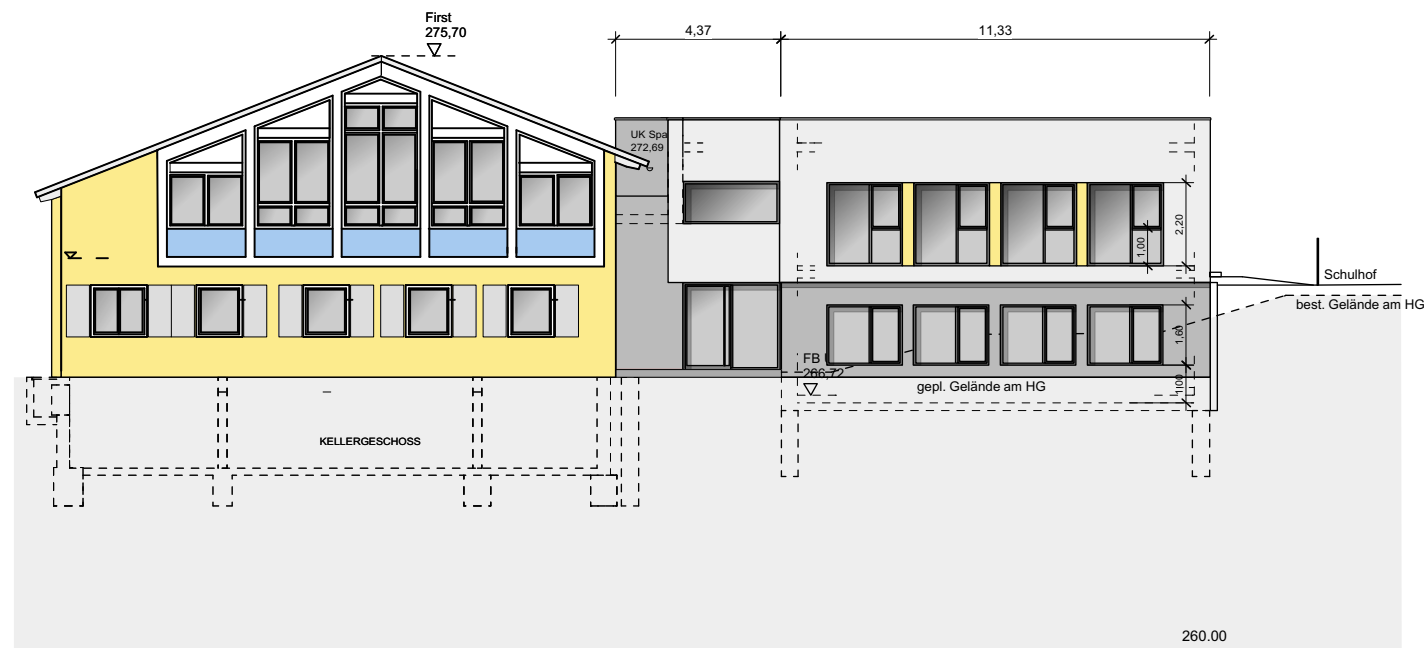
ANSICHT SÜD
